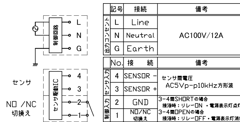
結線図
